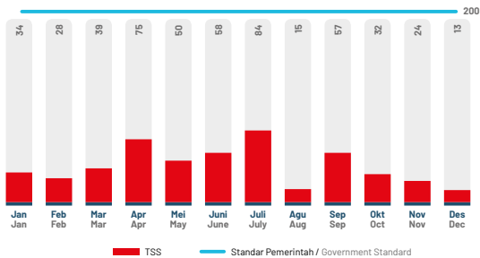
Rata-Rata Kandungan Padatan Tersuspensi pada Efluen BIB Tahun 2021 (mg/L) BIB's Average Suspended Solid Content in Effluent in 2021 (mg/L)
