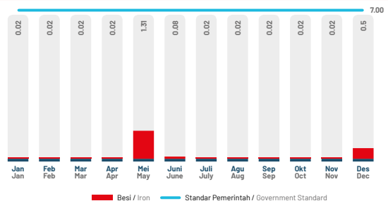
Kandungan Besi pada Efluen BIB Tahun 2021 (mg/L) BIB's Iron Content in Effluent in 2021 (mg/L)
